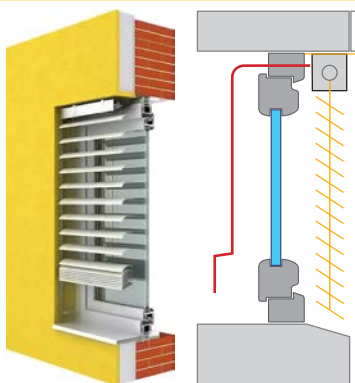
таванен монтаж
