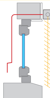
стенен монтаж
