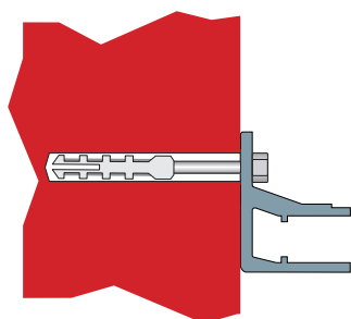
Монтаж в стена
